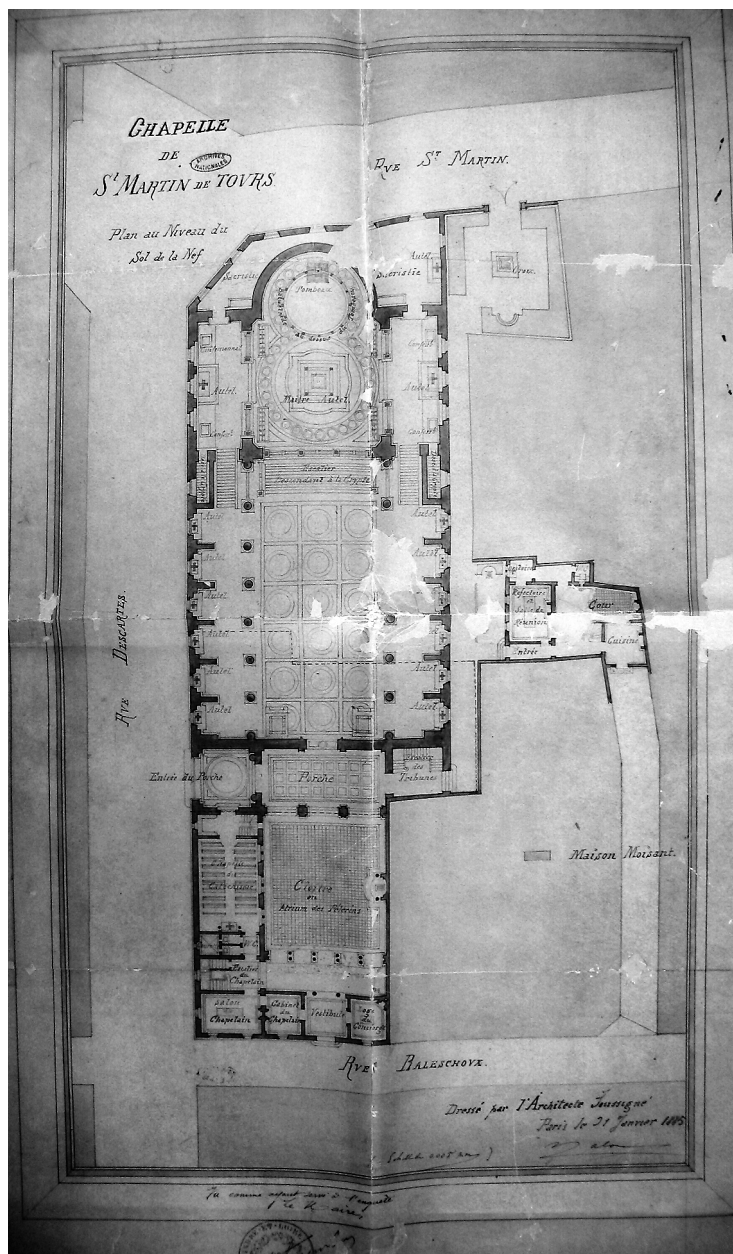
Fig. 4 : La chapelle de Saint-Martin (plan de Laloux, janvier 1885).
