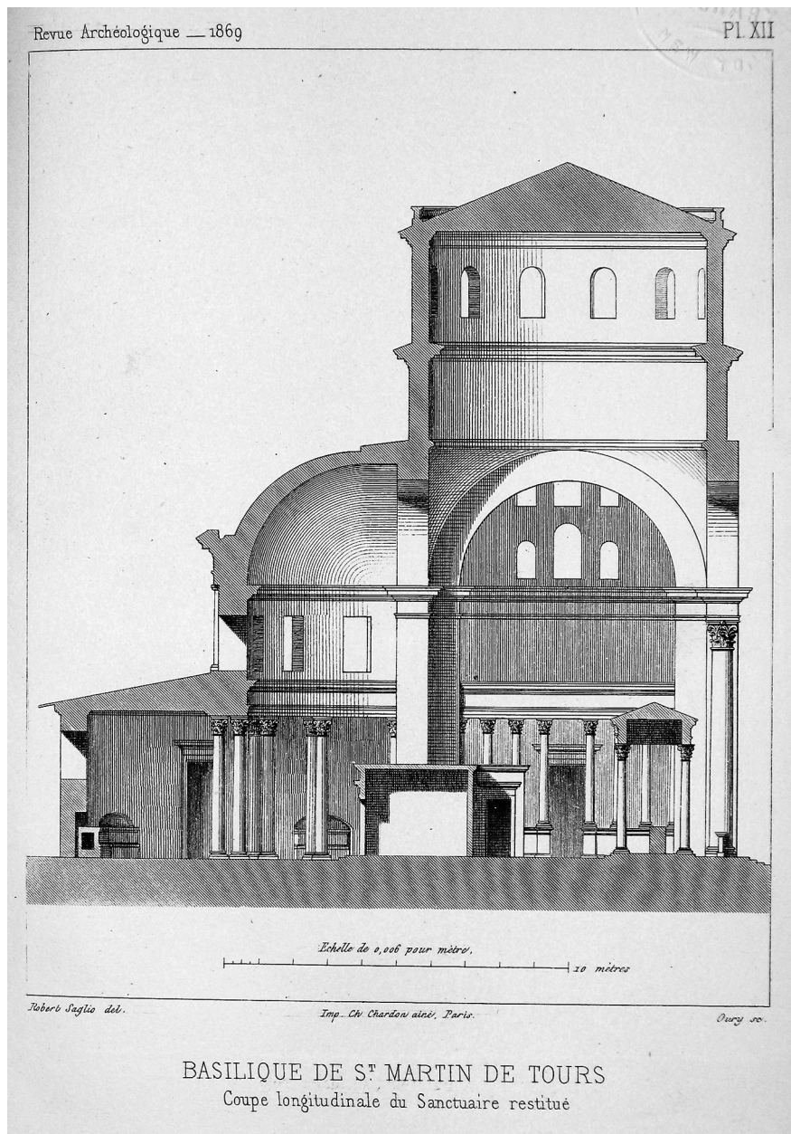
Fig. 3 : Restitution Quicherat ( Revue archéologique , 1869).
